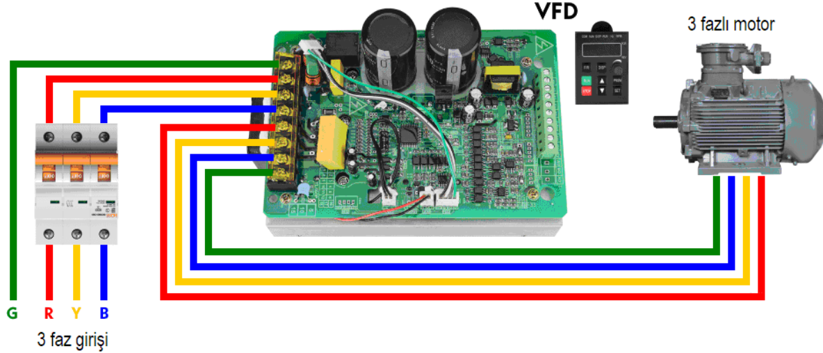
Şekil 1. Elektrik motoru için deęiřken frekanslı sürücü (VFD) baęlantı řeması
