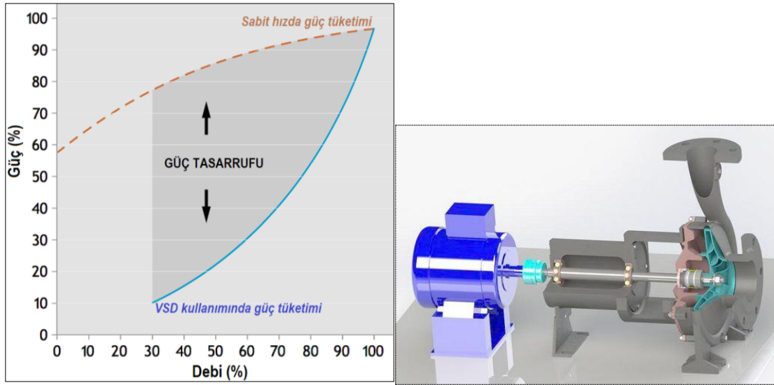
Şekil 6. VFD kullanımı ile güç tasarrufu
